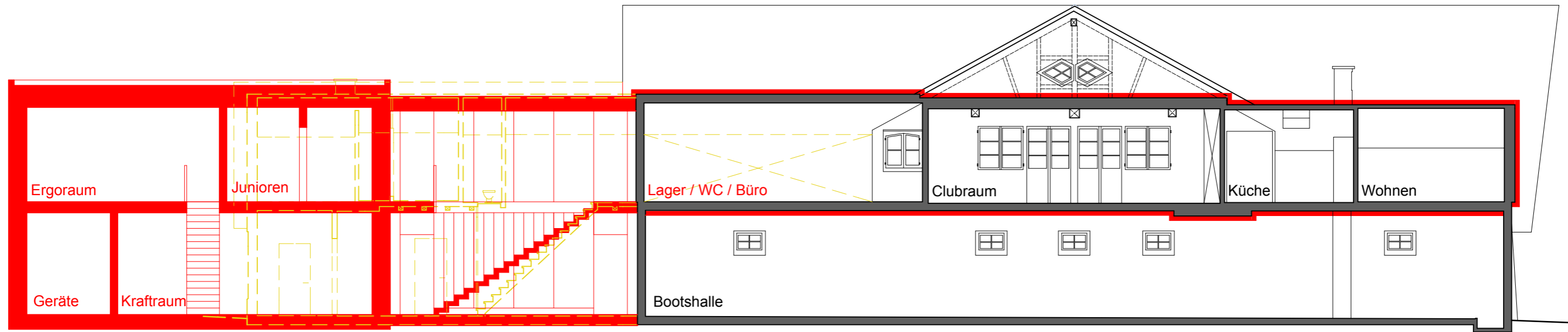
Längsschnitt C-C
